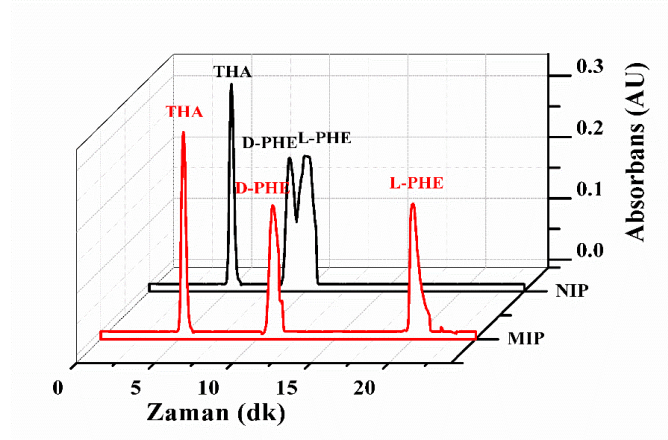
Resim 1. Baskılanmamış (NIP)-(boş) kolonda fenilalaninin çakıştırılmış elektrogramda enantiyomerik ayırımı: uygulanan voltaj: 10 kV, basınç: 0 mbar, konsantrasyon: 0.5 mg/mL, dalgaboyu: 200 nm; (ACN %50 - pH 7 %50)
